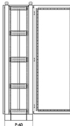
VISTA SEM TAMPA LATERAL PORTA ABERTA
