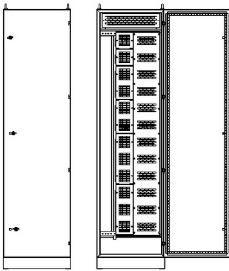
VISTA TRASEIRA PORTA ABERTA
